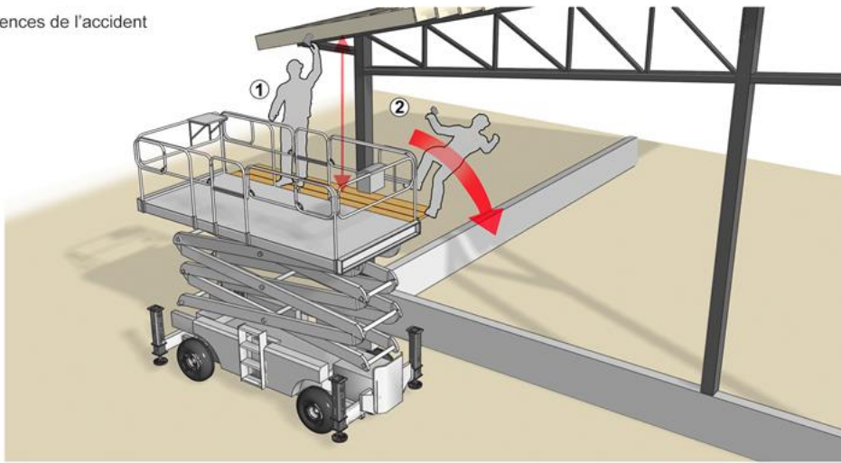
Plateforme sans les accessoires sécuritaires
